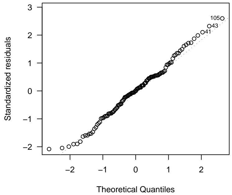
Normal Q-Q
