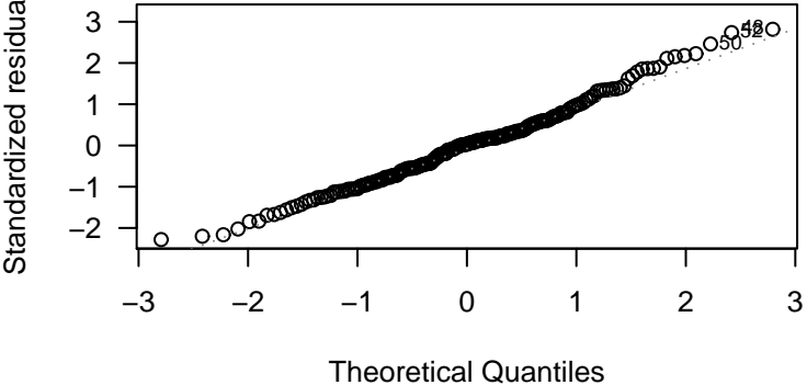
Normal Q-Q
