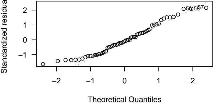
Normal Q-Q
