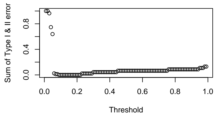
(1-Sens.) + (1-Spec.)
