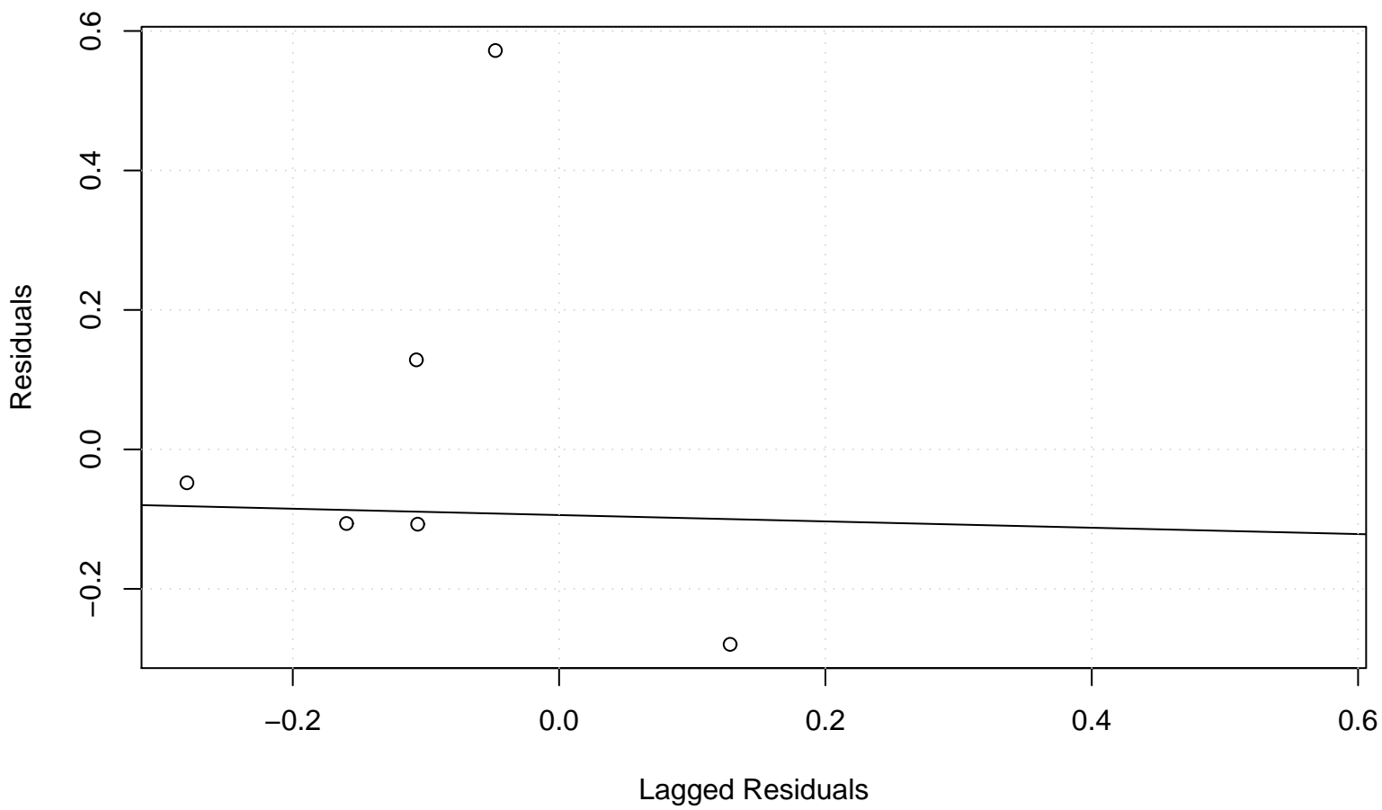
Lag plot
