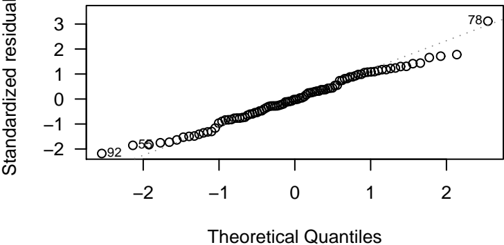
Normal Q-Q
