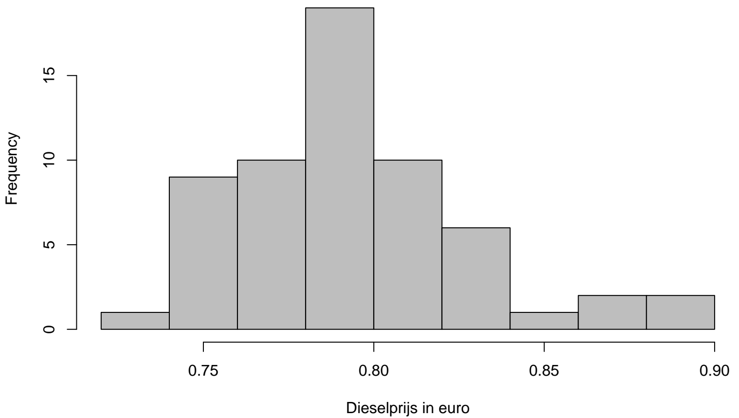
Histogram dieselprijs
