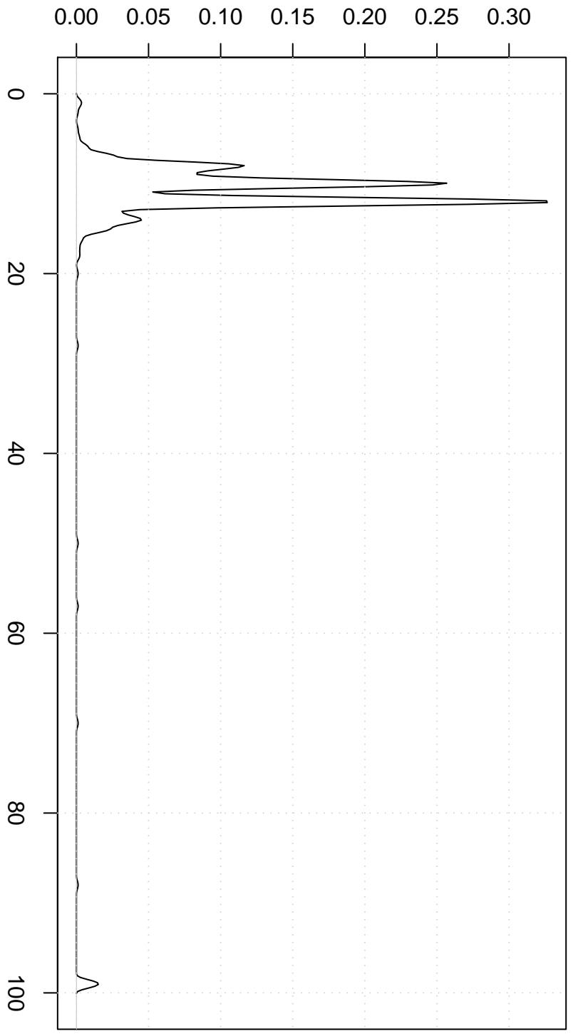
Cosine Kernel
