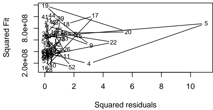
Sq.Resid vs. Sq.Fit
