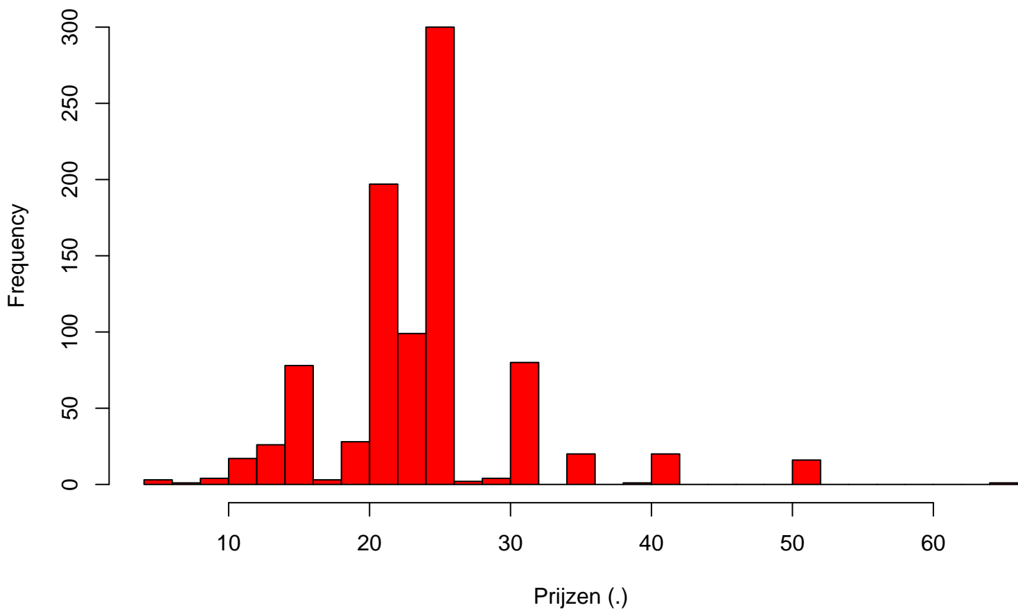
Histogram Maximumprijzen
