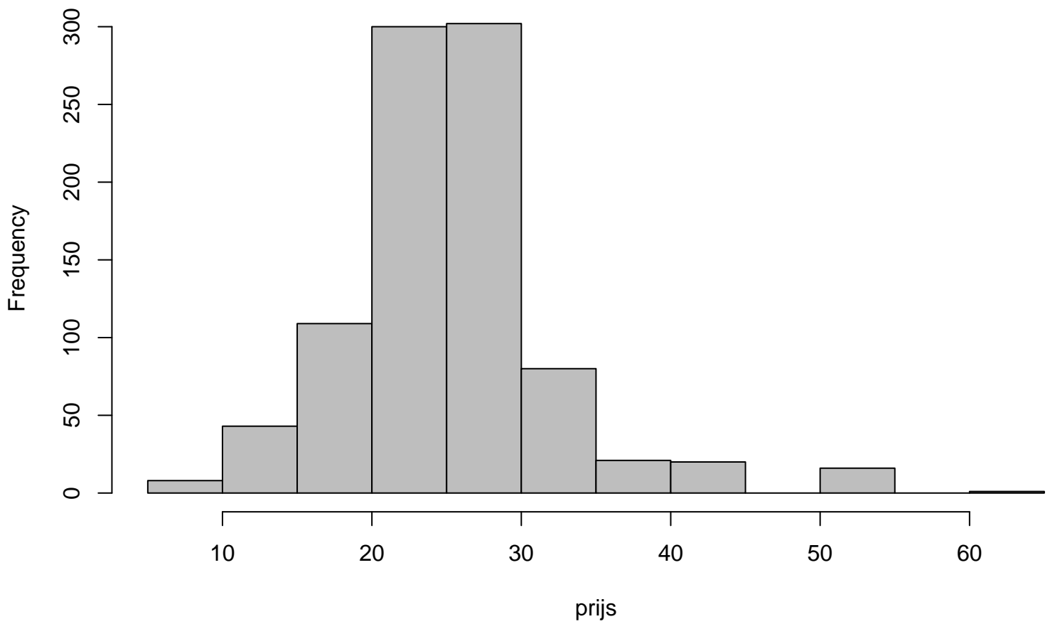
Histogram maximumprijs van een show
