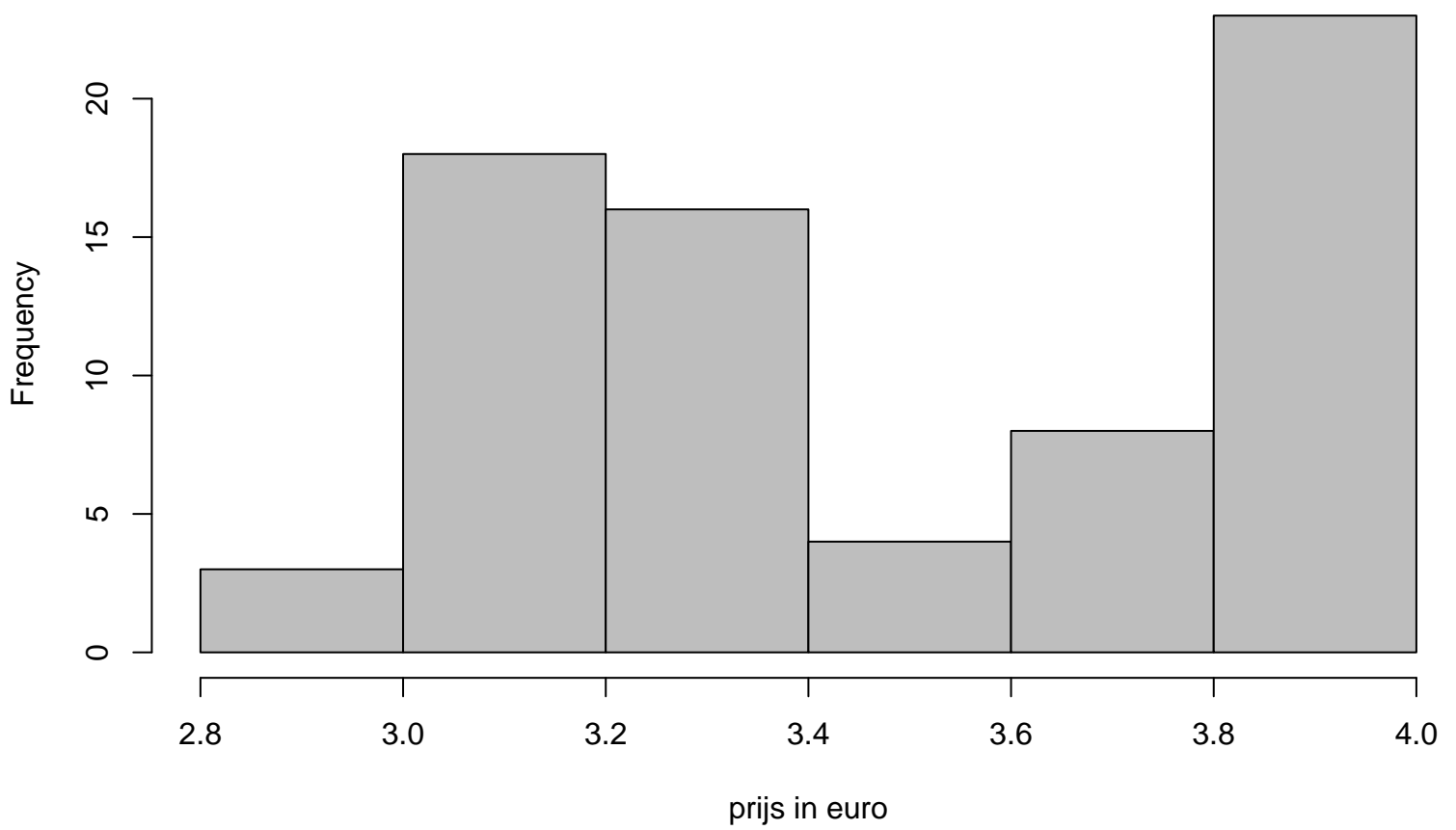
Histogram frequentietabel
