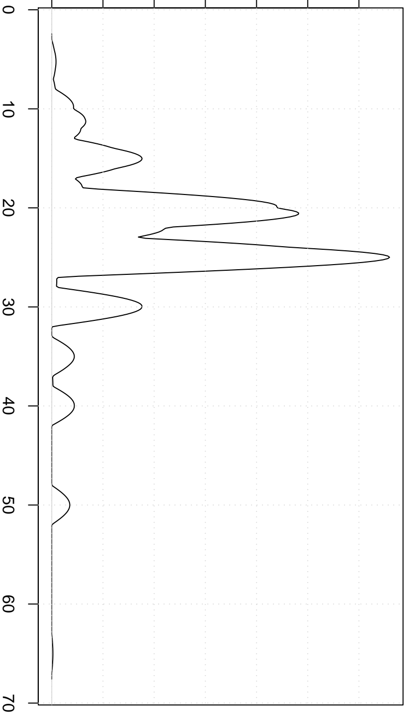
Optcosine Kernel
