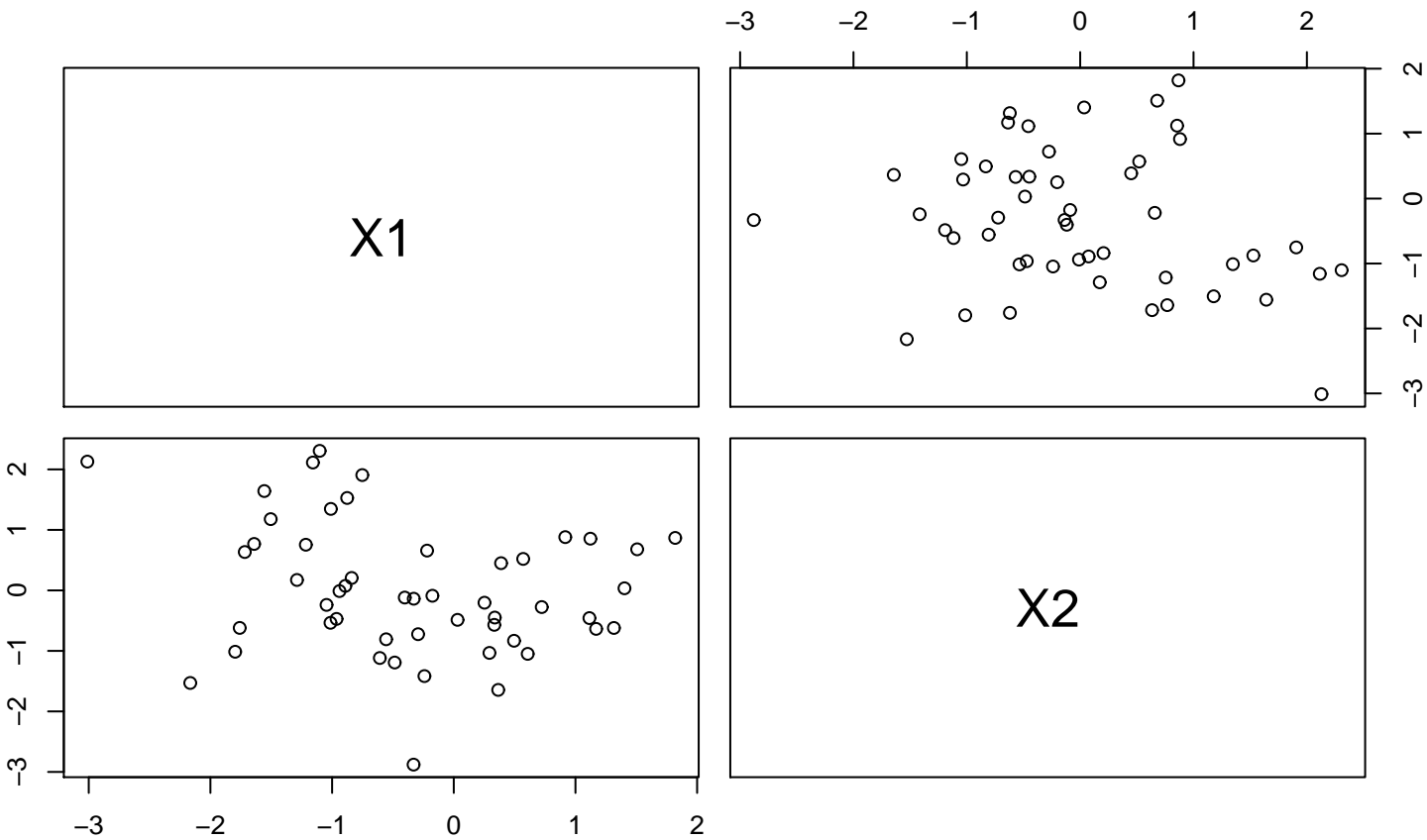
pairs plot
