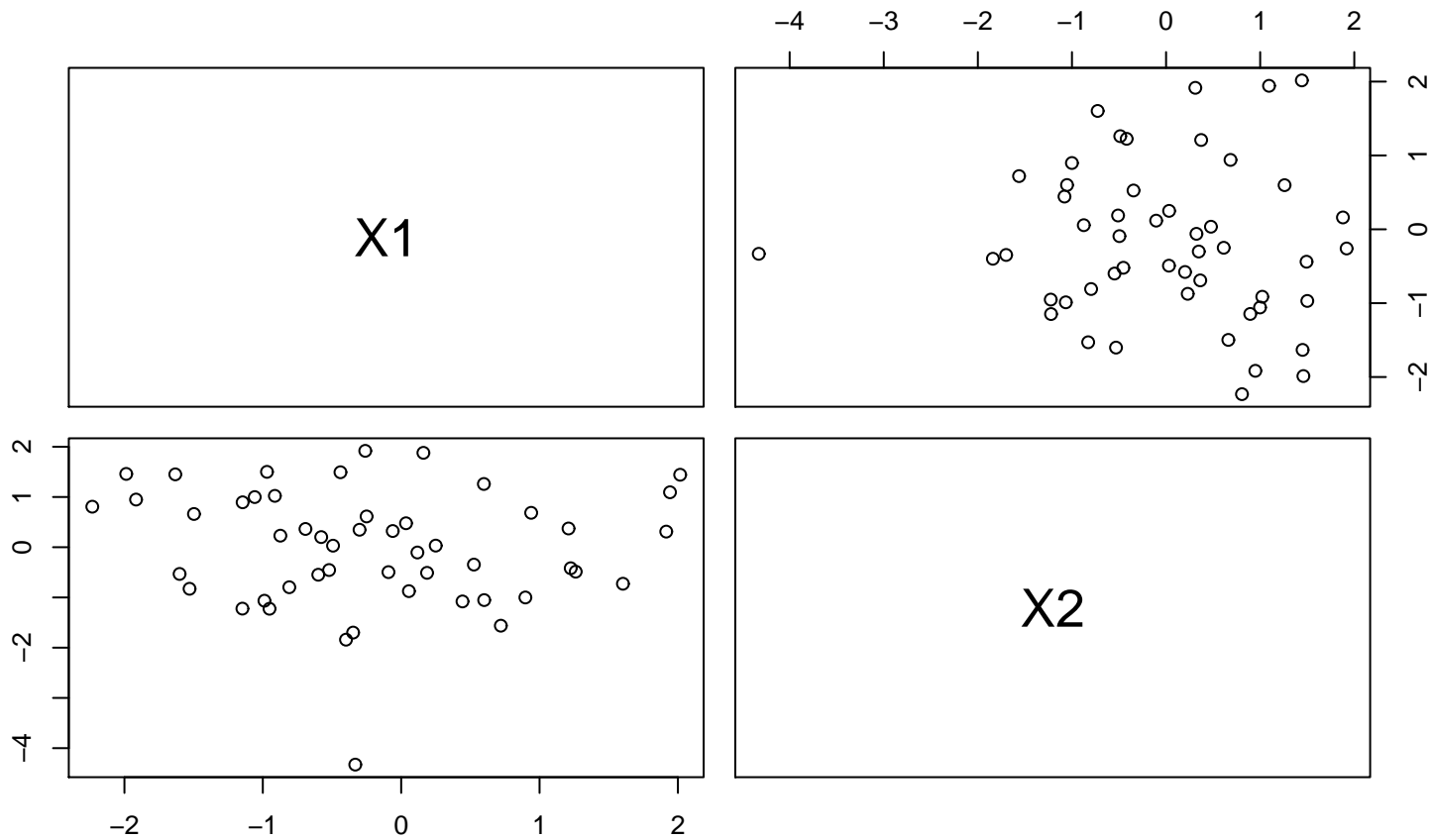
pairs plot
