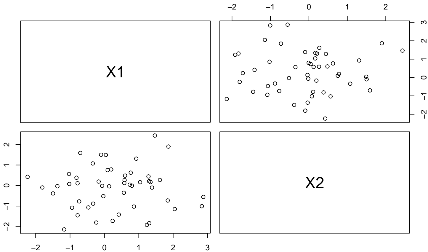
pairs plot
