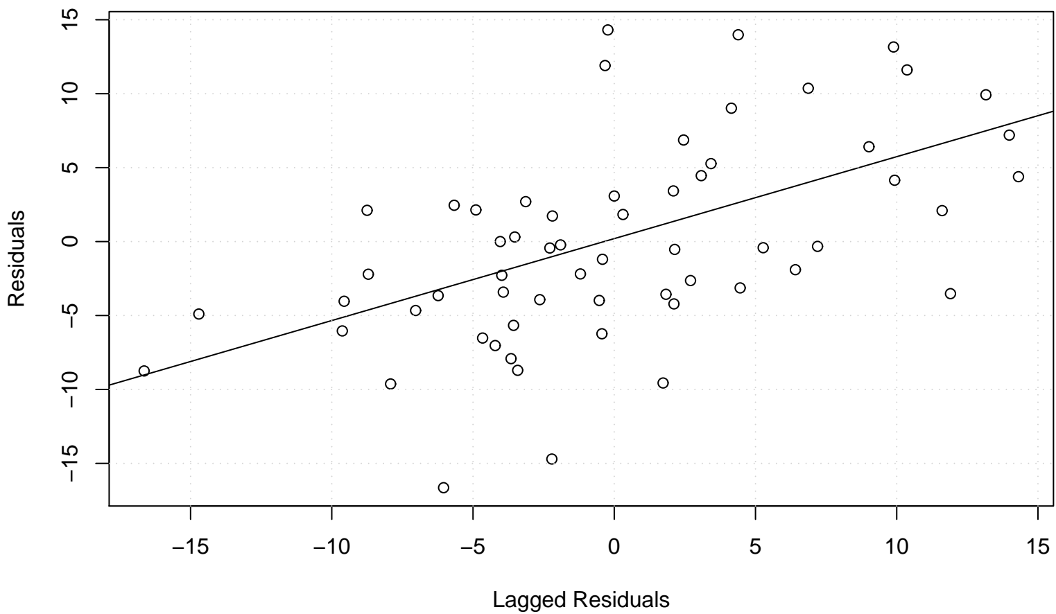
Lag plot
