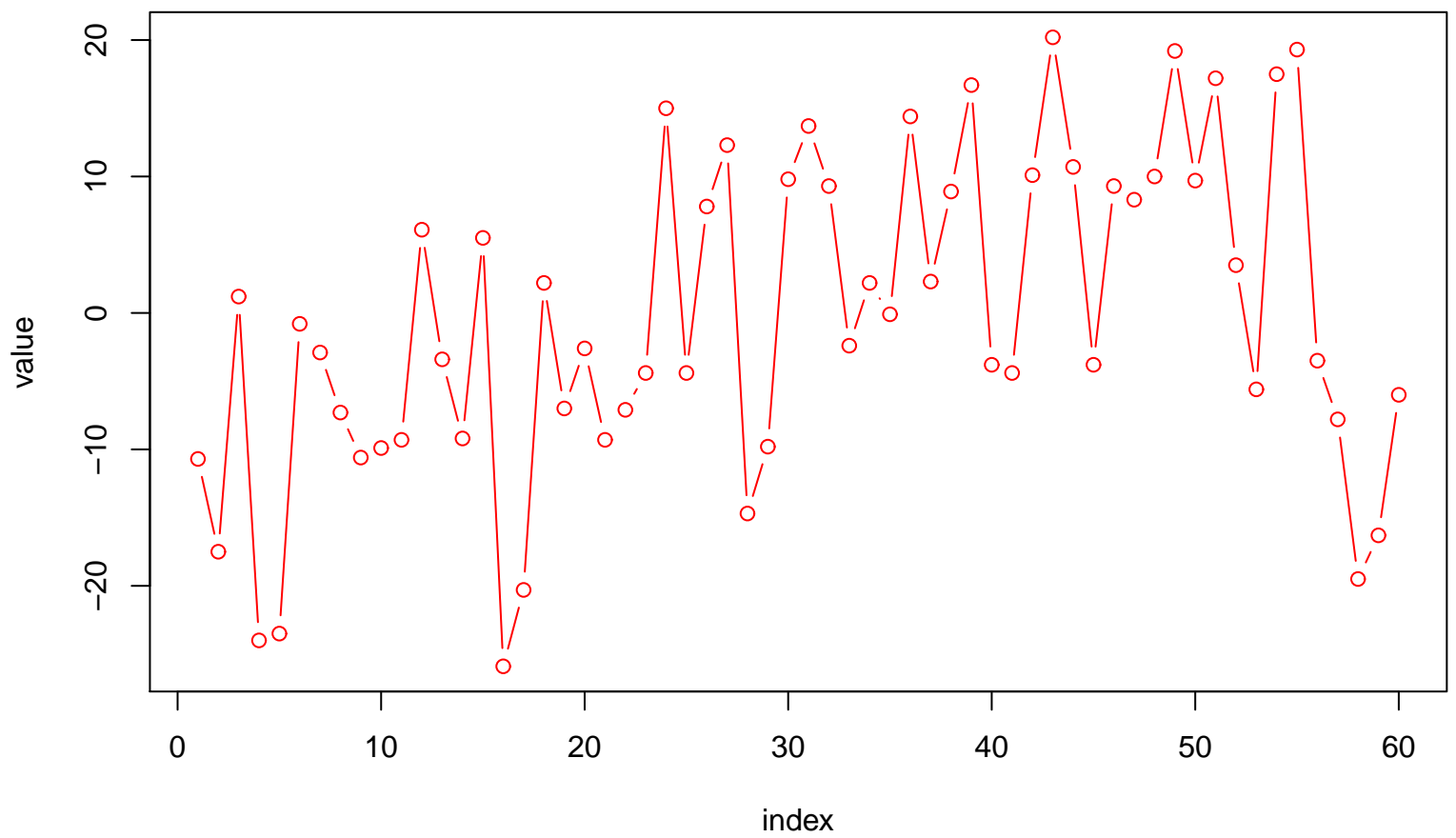
e[t] voor Y[t] = 118.718 + e[t]
