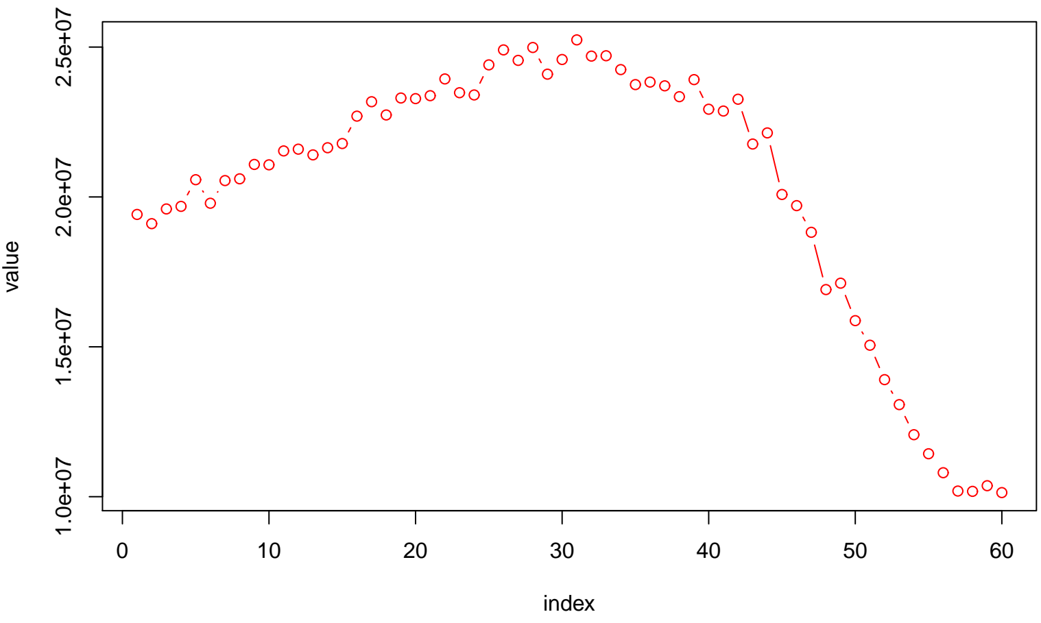
Industrial production * werkloosheid
