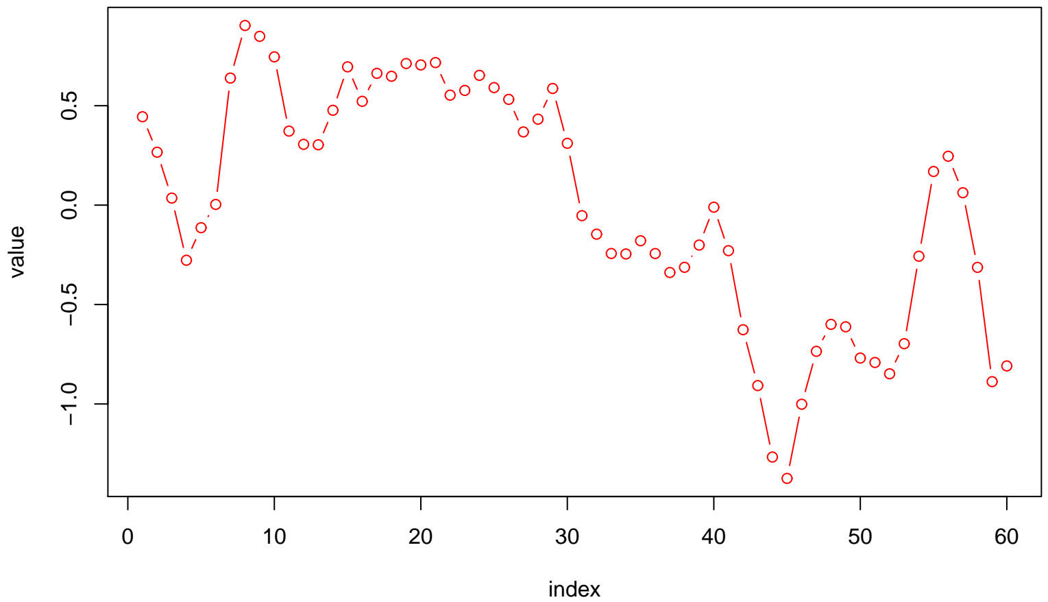
e[t] bij model 1. Y[t] = c + b X[t] + e
