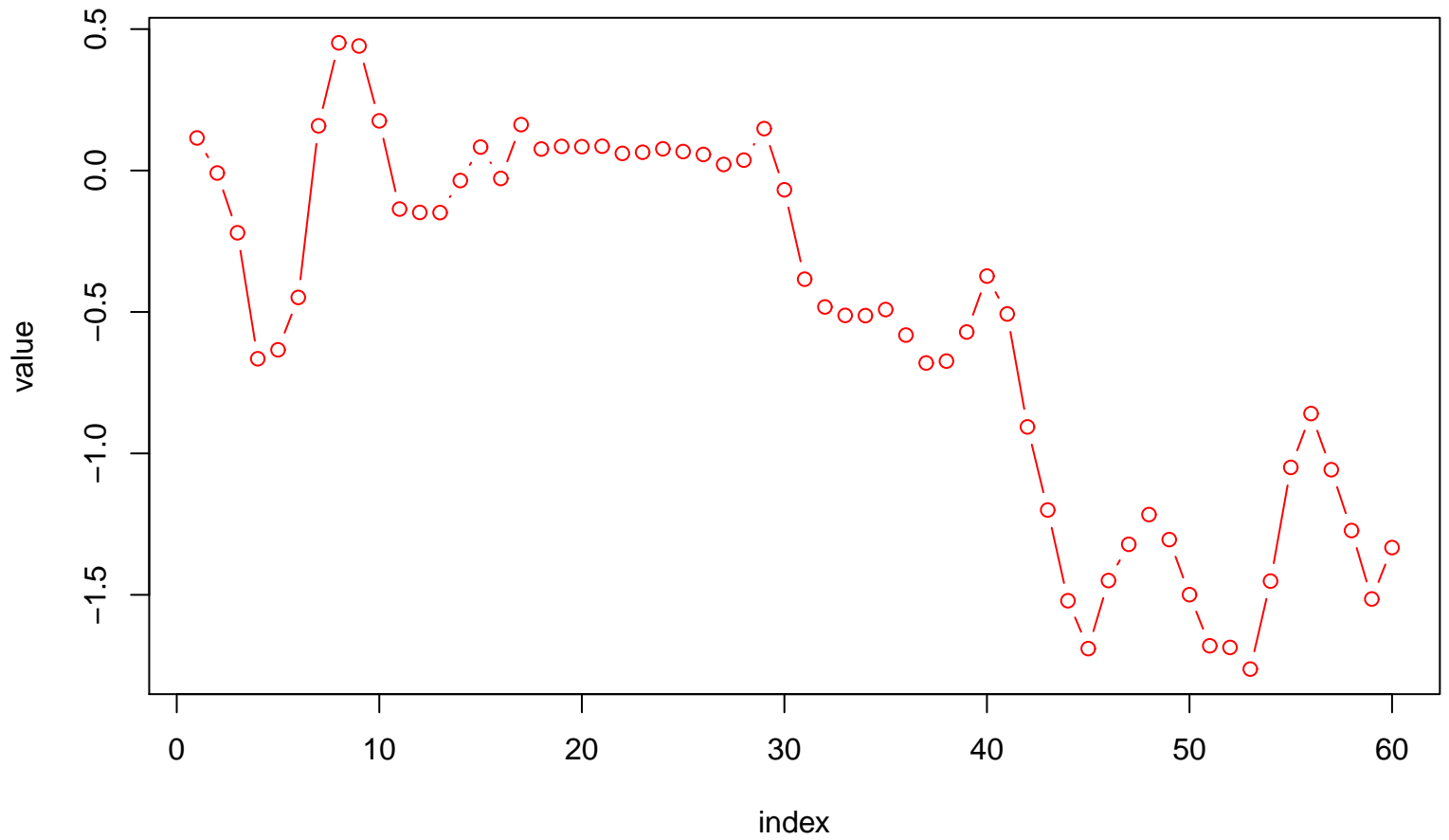
e bij model 3. Y[t] = c + b \ln X[t] + e
