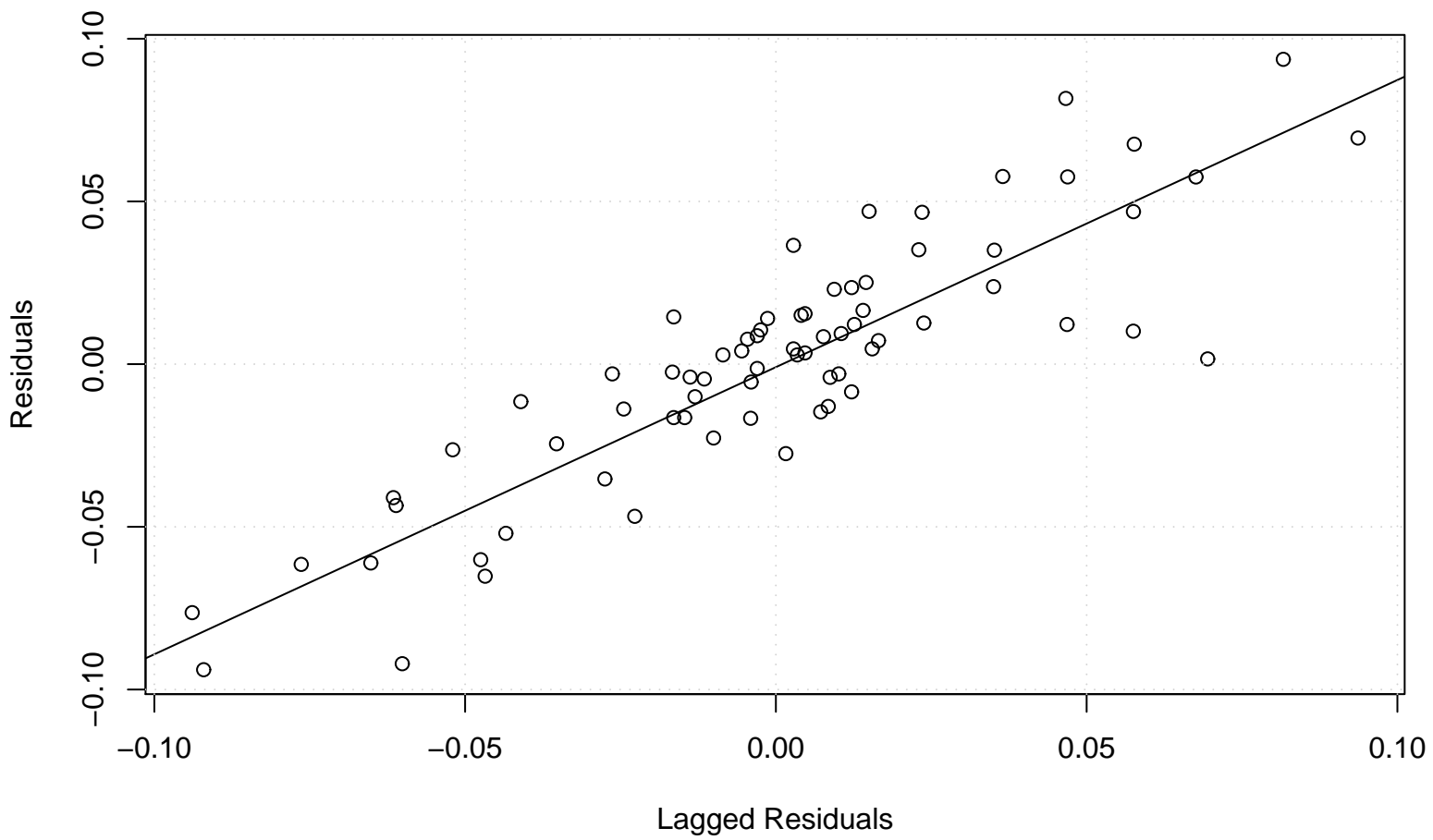
Lag plot
