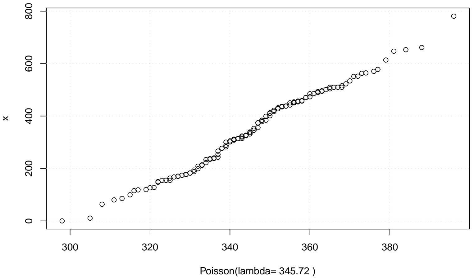
QQ plot (Poisson)
