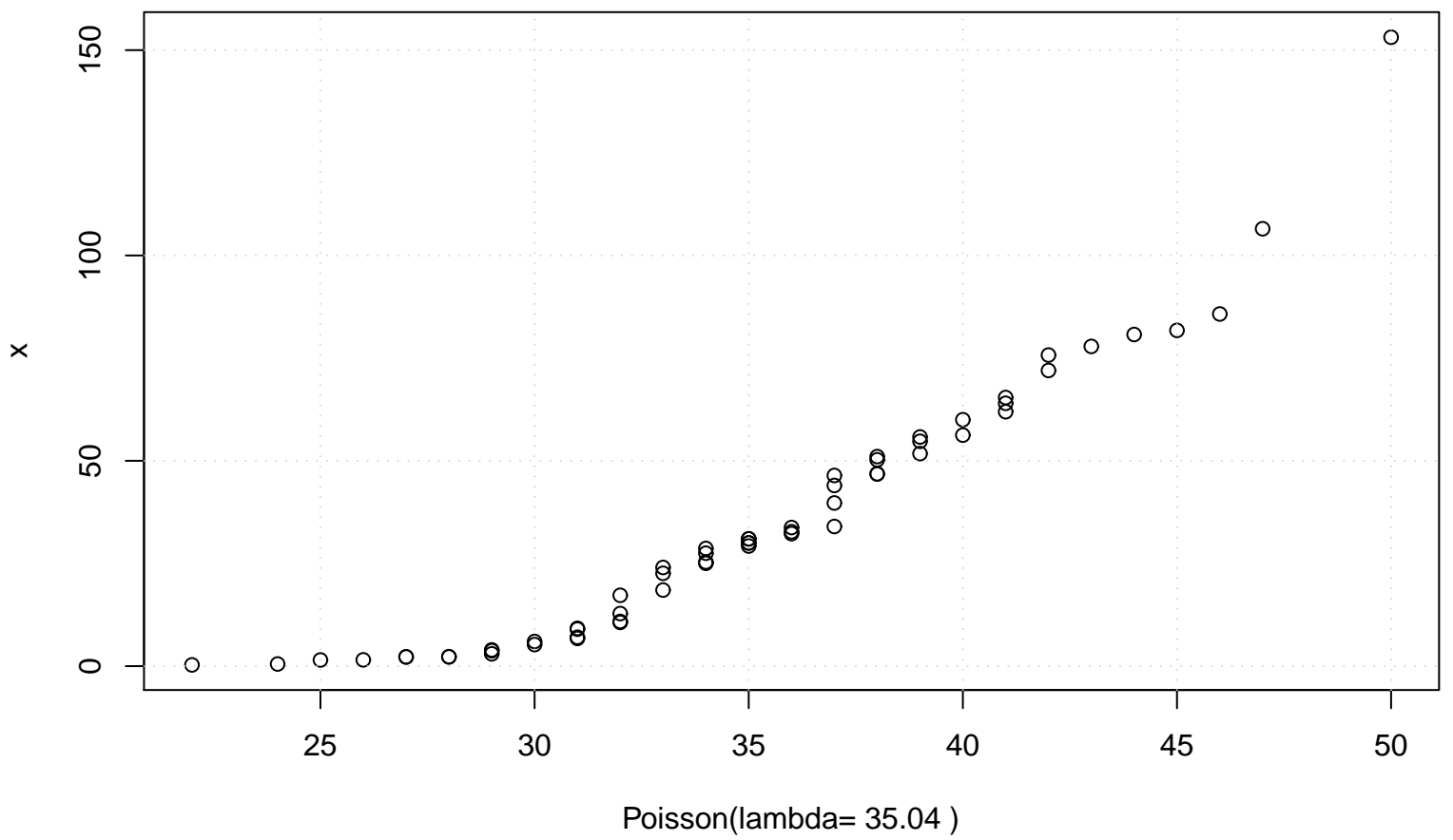
QQ plot (Poisson)
