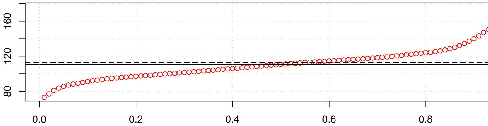
Harrell–Davis Quantiles
