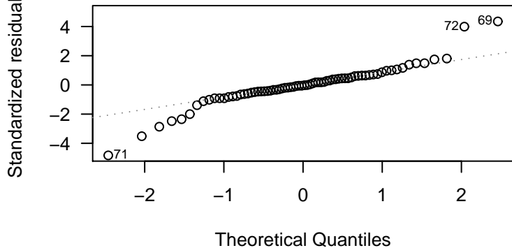
Normal Q-Q
