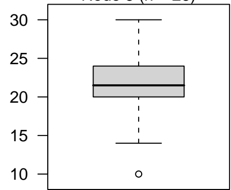
Node 5 (n = 26)
