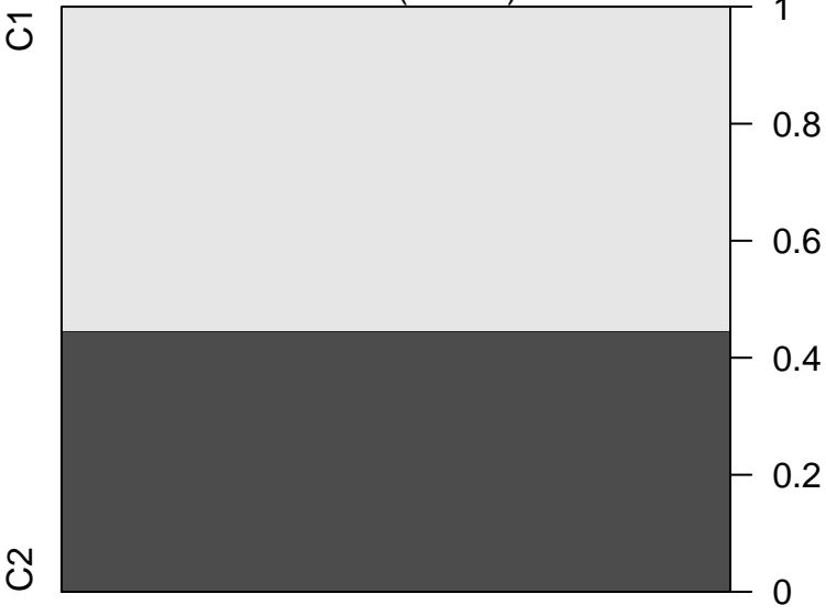
Node 2 (n = 56)
