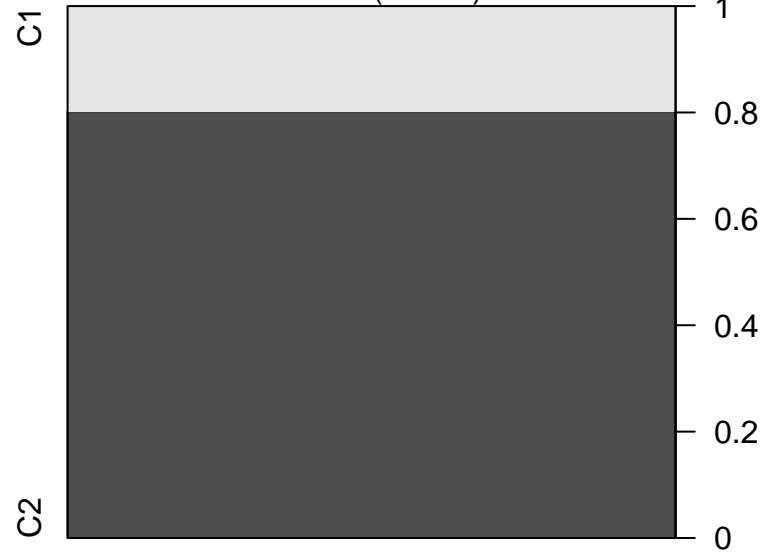
Node 3 (n = 81)
