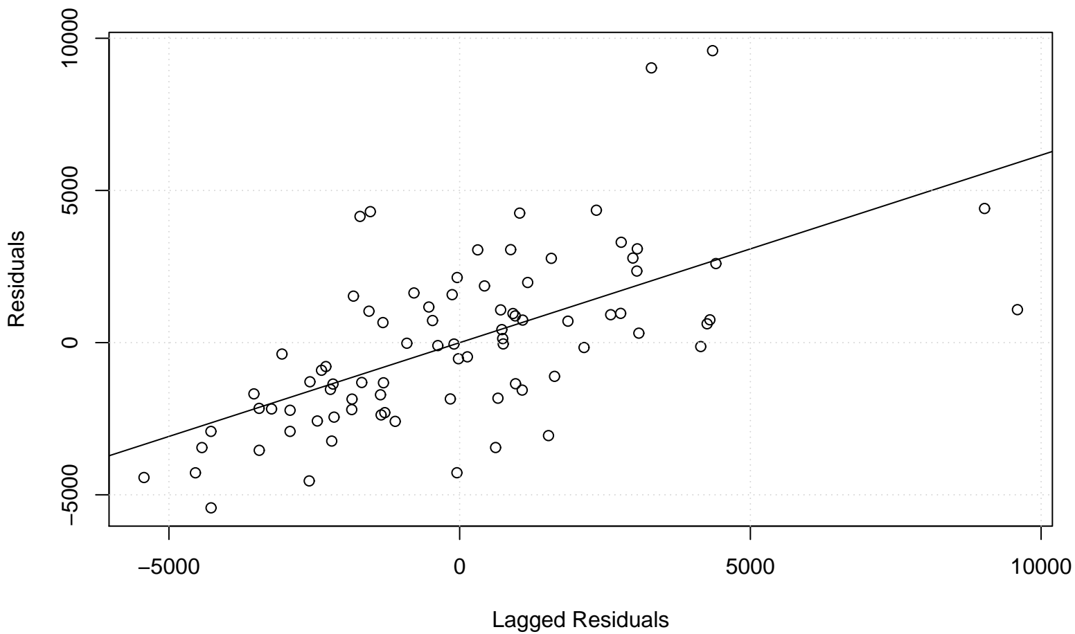
Lag plot
