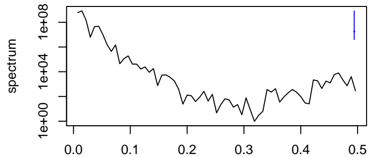
Trend
