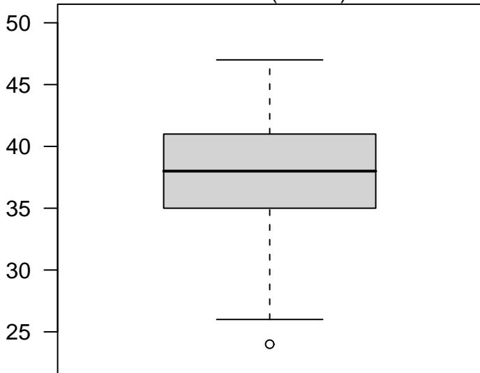
Node 2 (n = 54)
