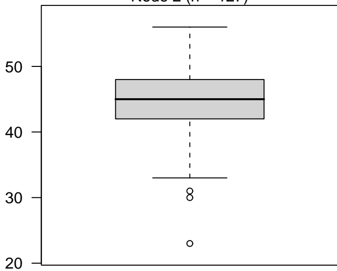
Node 2 (n = 127)
