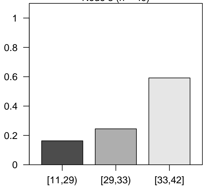
Node 3 (n = 49)
