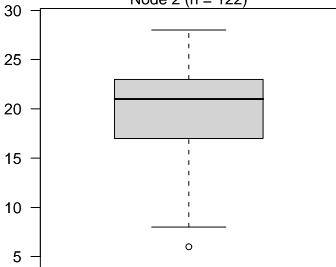
Node 2 (n = 122)
