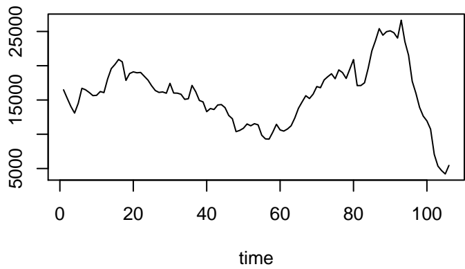
d=0, D=1
