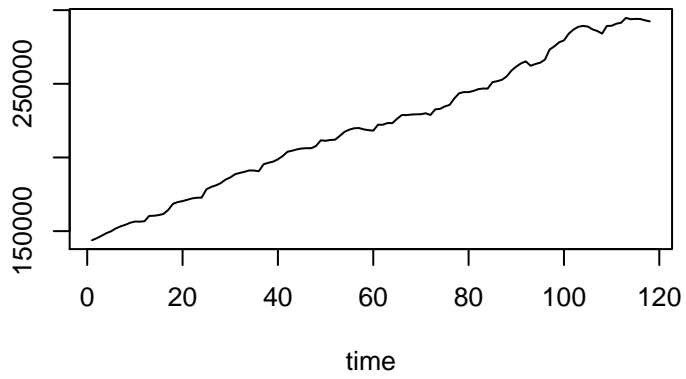
d=0, D=0
