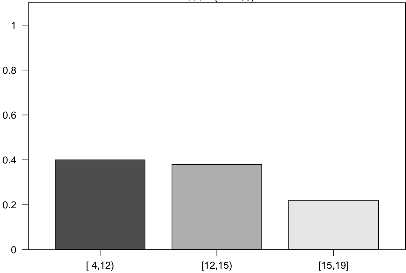
Node 1 (n = 150)
