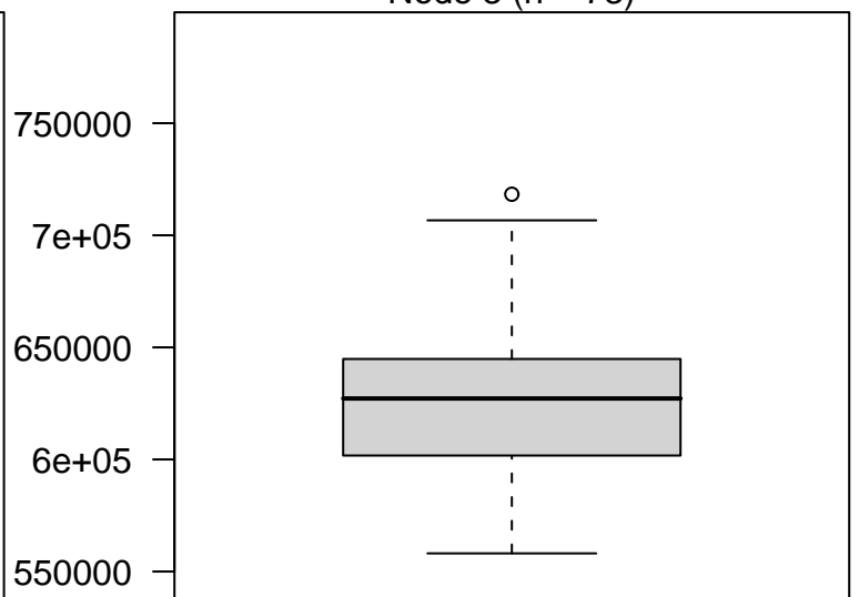
Node 3 (n = 73)
