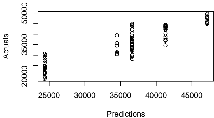
Actuals versus Predictions
