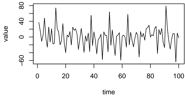
d=1, D=0
