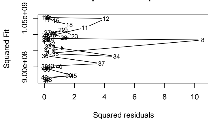
Sq.Resid vs. Sq.Fit
