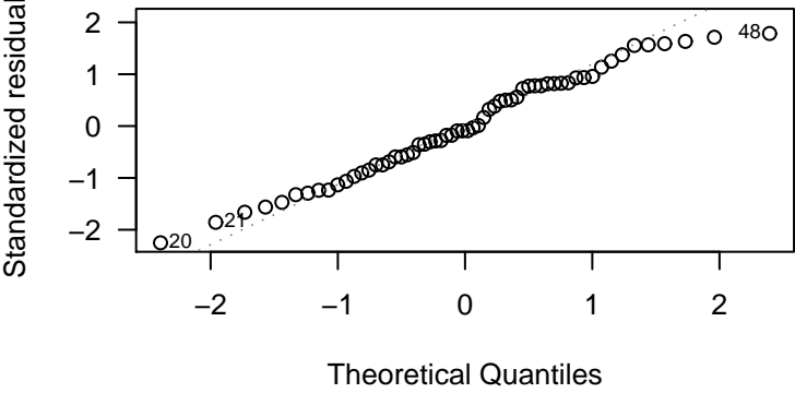
Normal Q-Q
