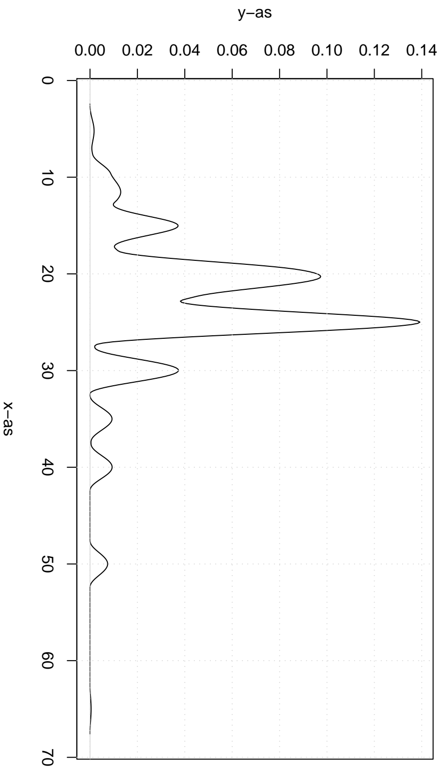
Cosine Kernel
