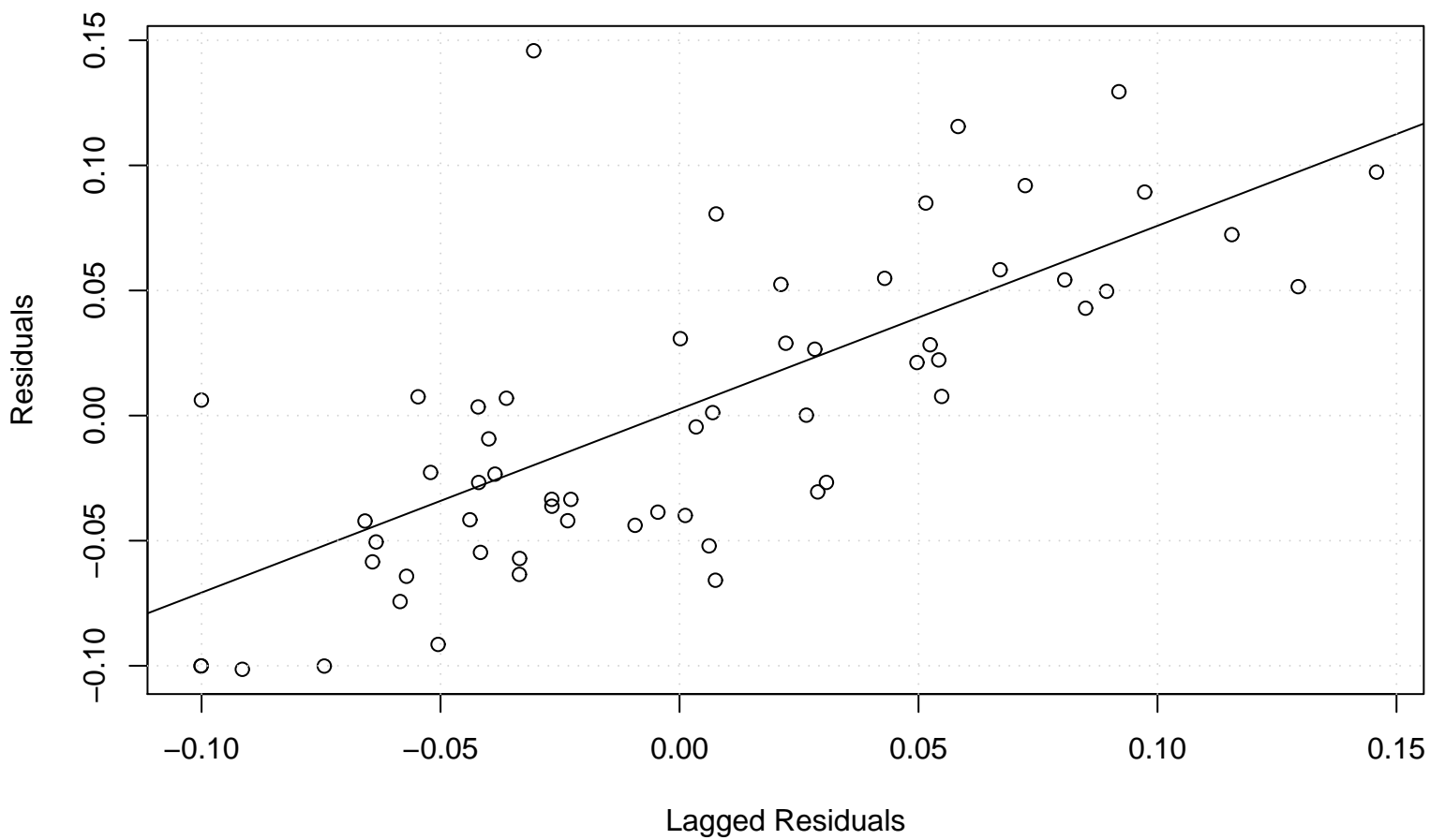
Lag plot
