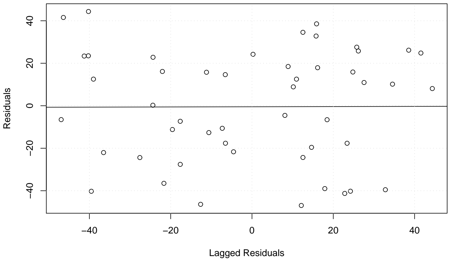
Lag plot
