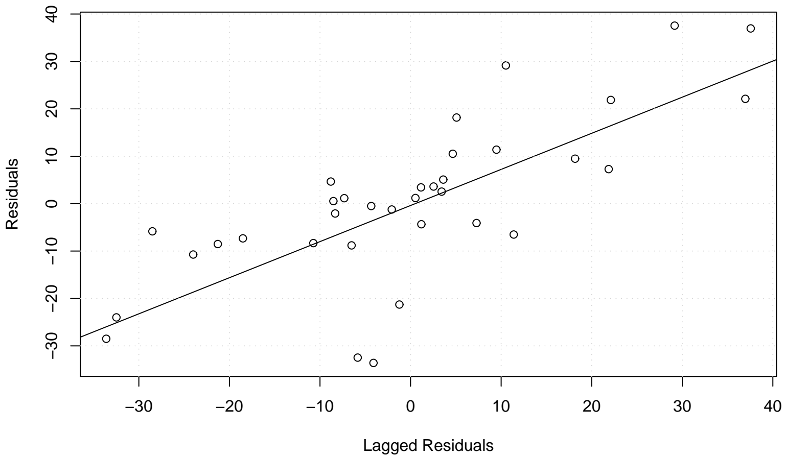
Lag plot
