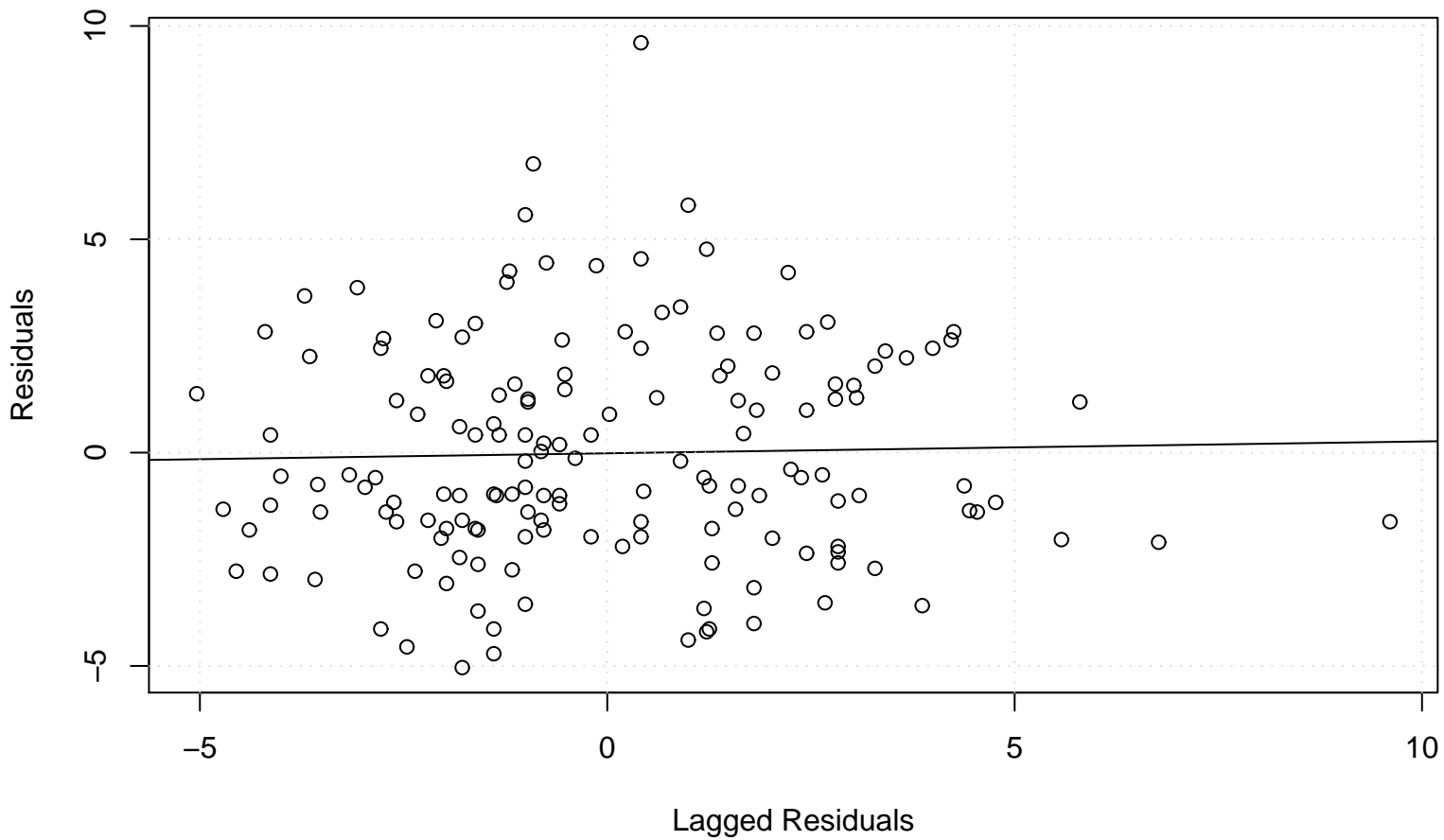
Lag plot
