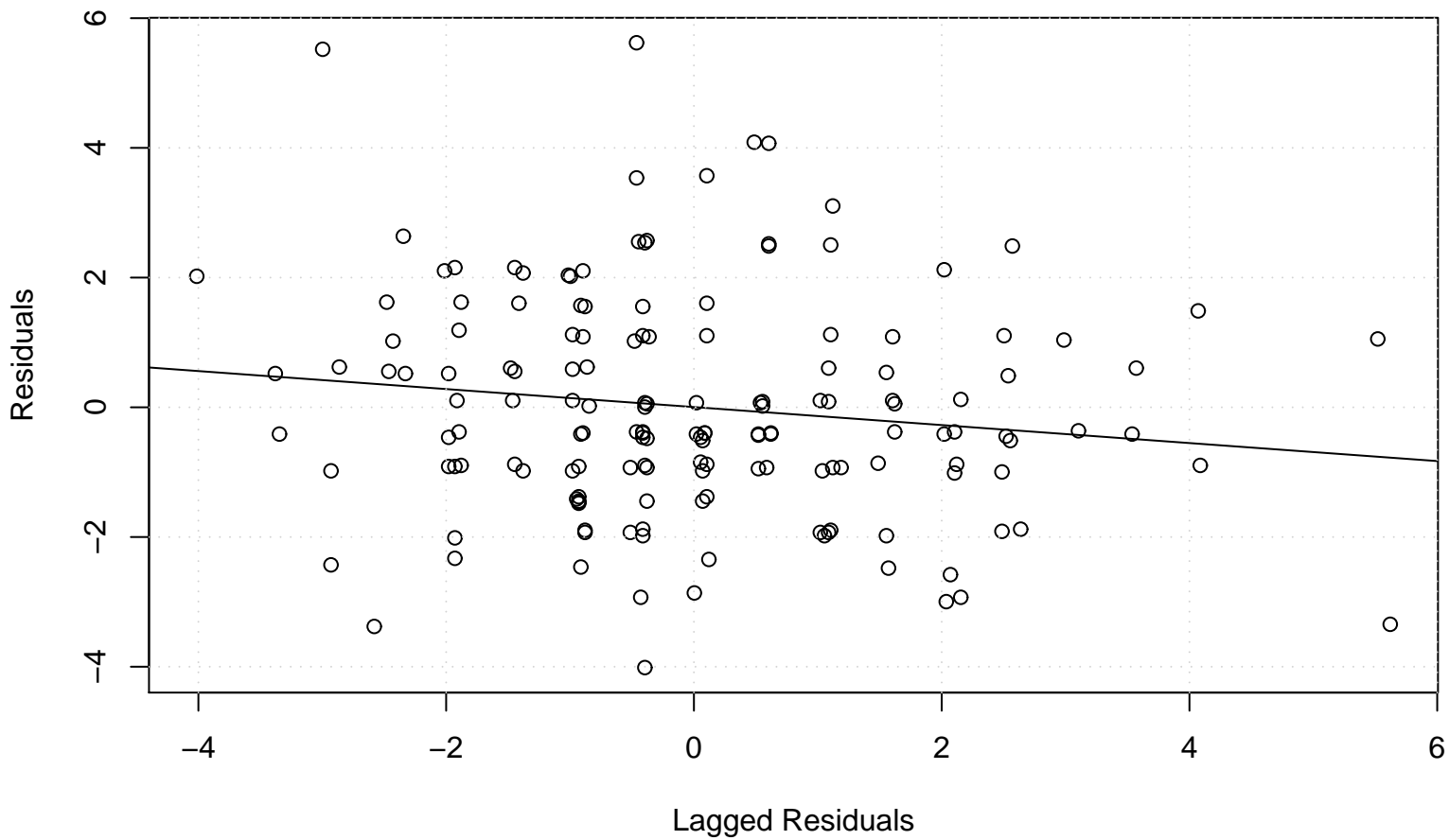
Lag plot
