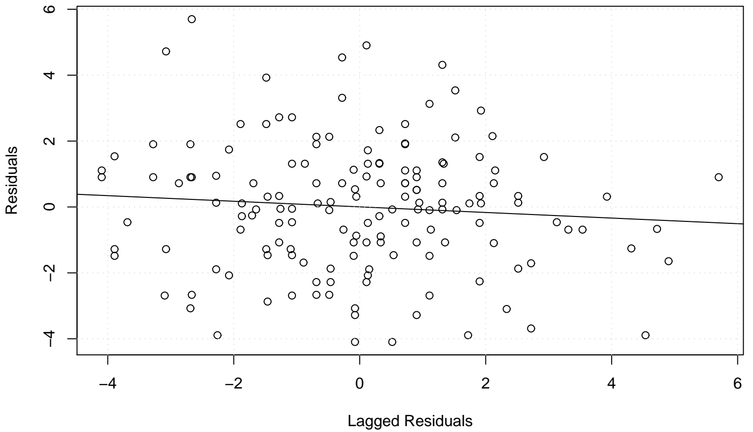
Lag plot
