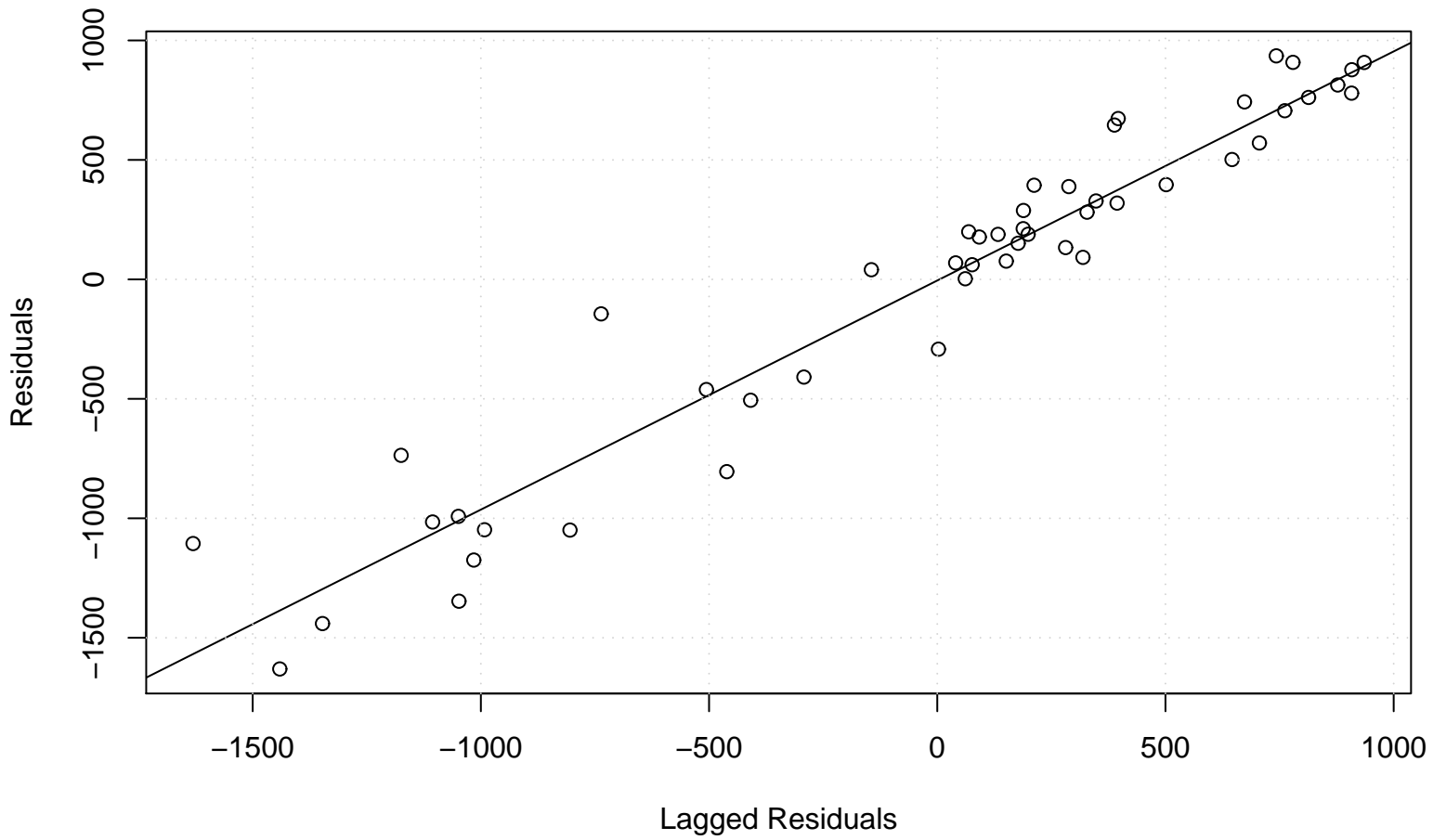
Lag plot
